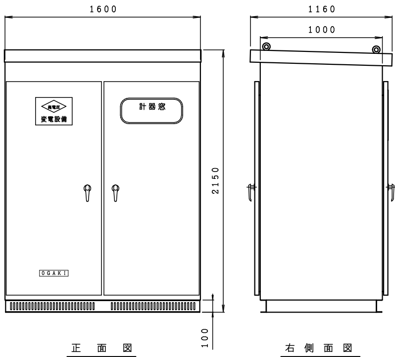
外形図
