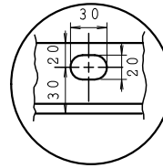
基礎穴詳細図
