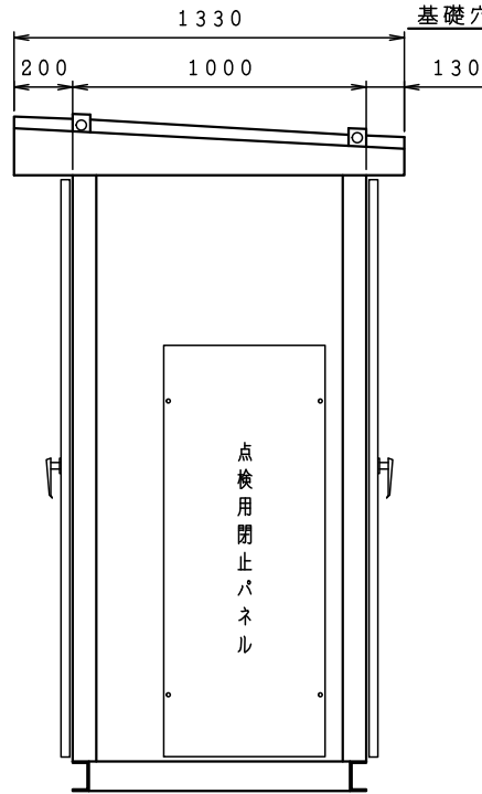
右側面図
