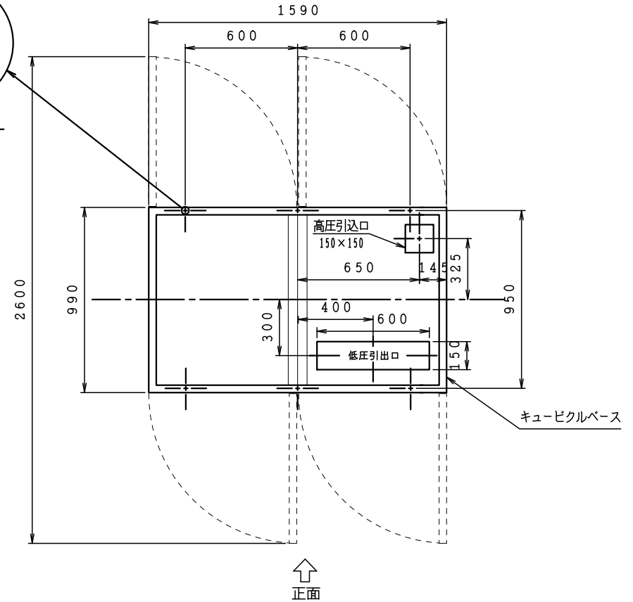
基礎穴詳細図
