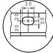
基礎穴詳細図
