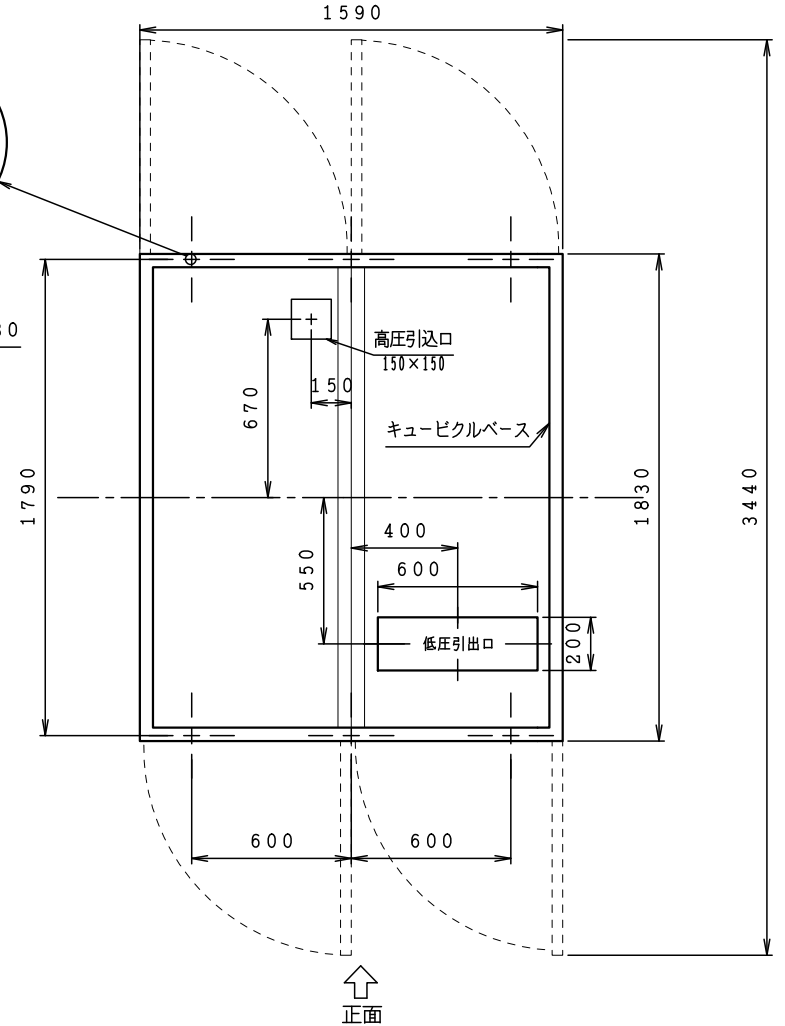
基礎図
