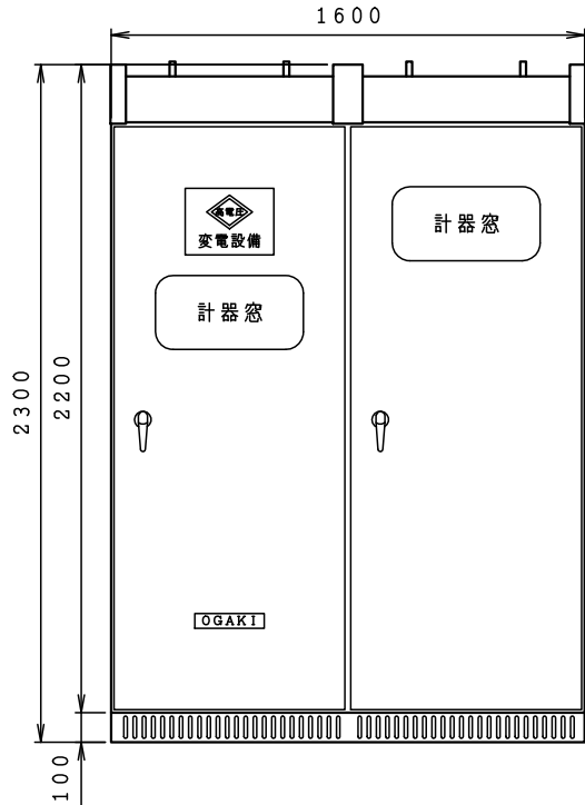
正面図
