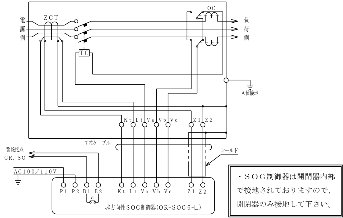
OAG-C5形高压気中開閉器
