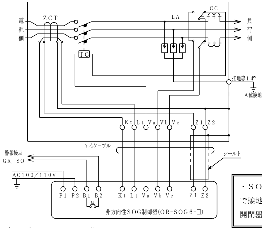
OAG-CL5形高圧気中開閉器
