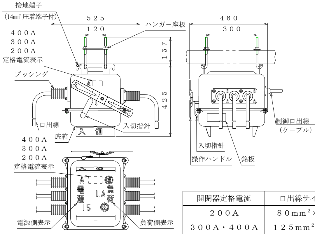
OAG-CL5形高圧気中開閉器
