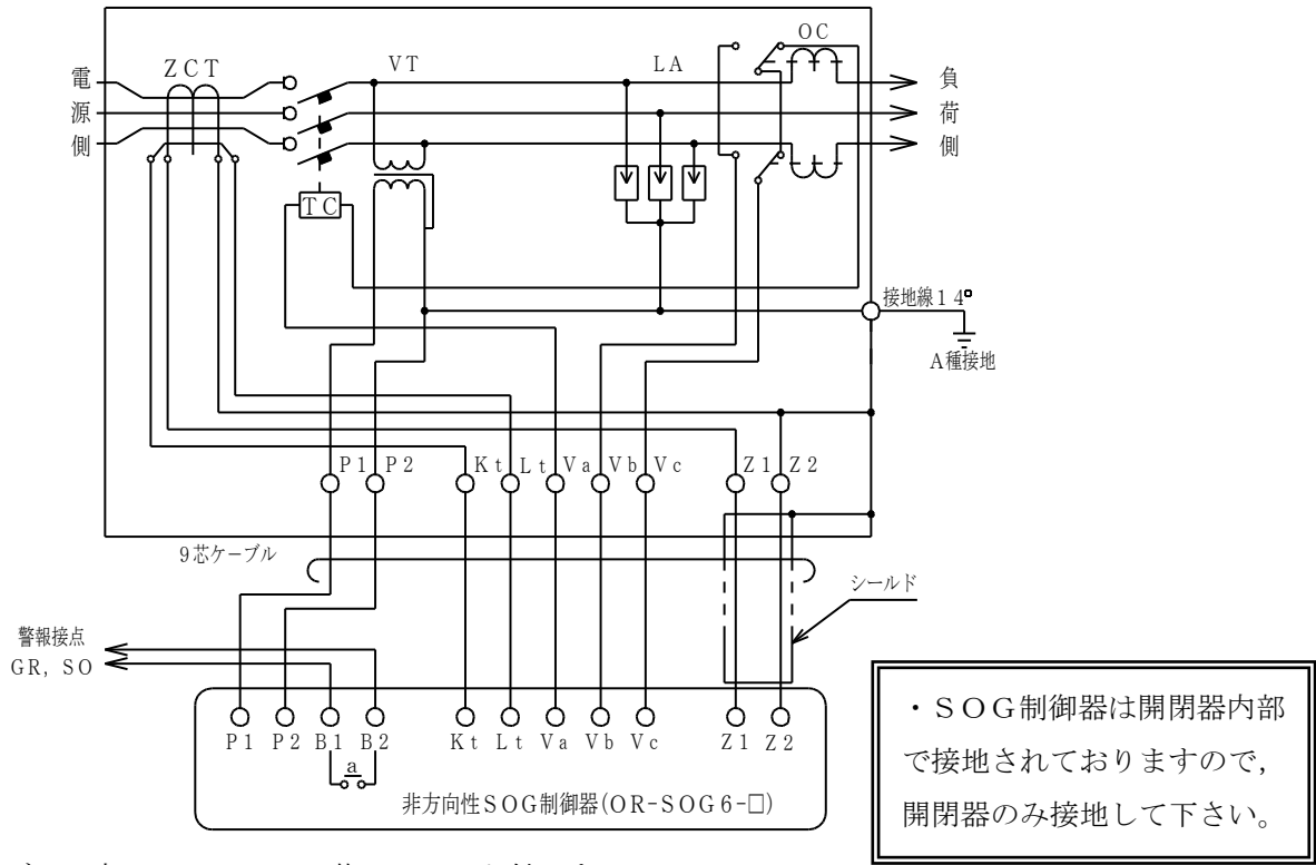
OAG-CPL5形高压気中開閉器
