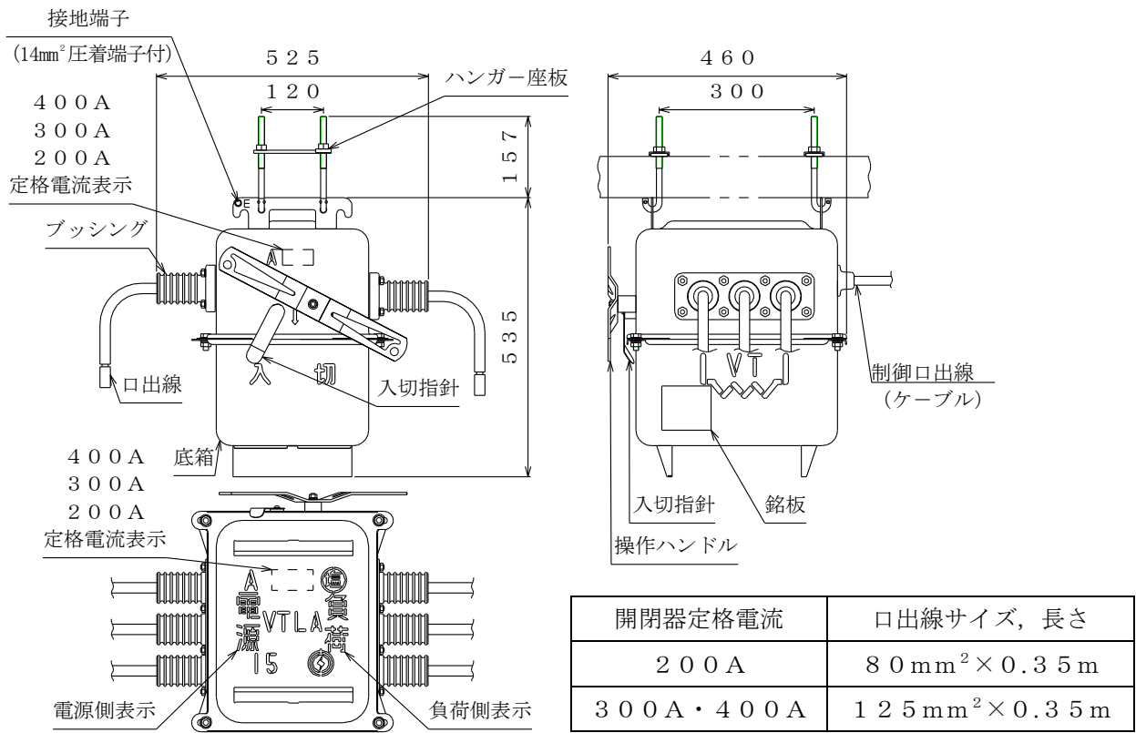
OAG-CPL5形高压気中開閉器
