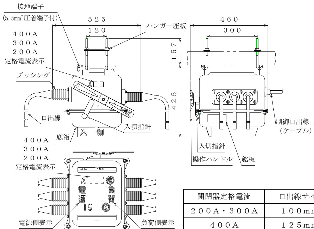
OAG-CK5形高圧気中開閉器
