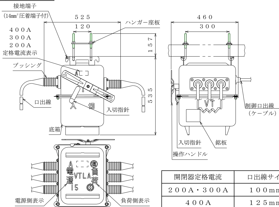
OAG-CPLK5形高圧気中開閉器
