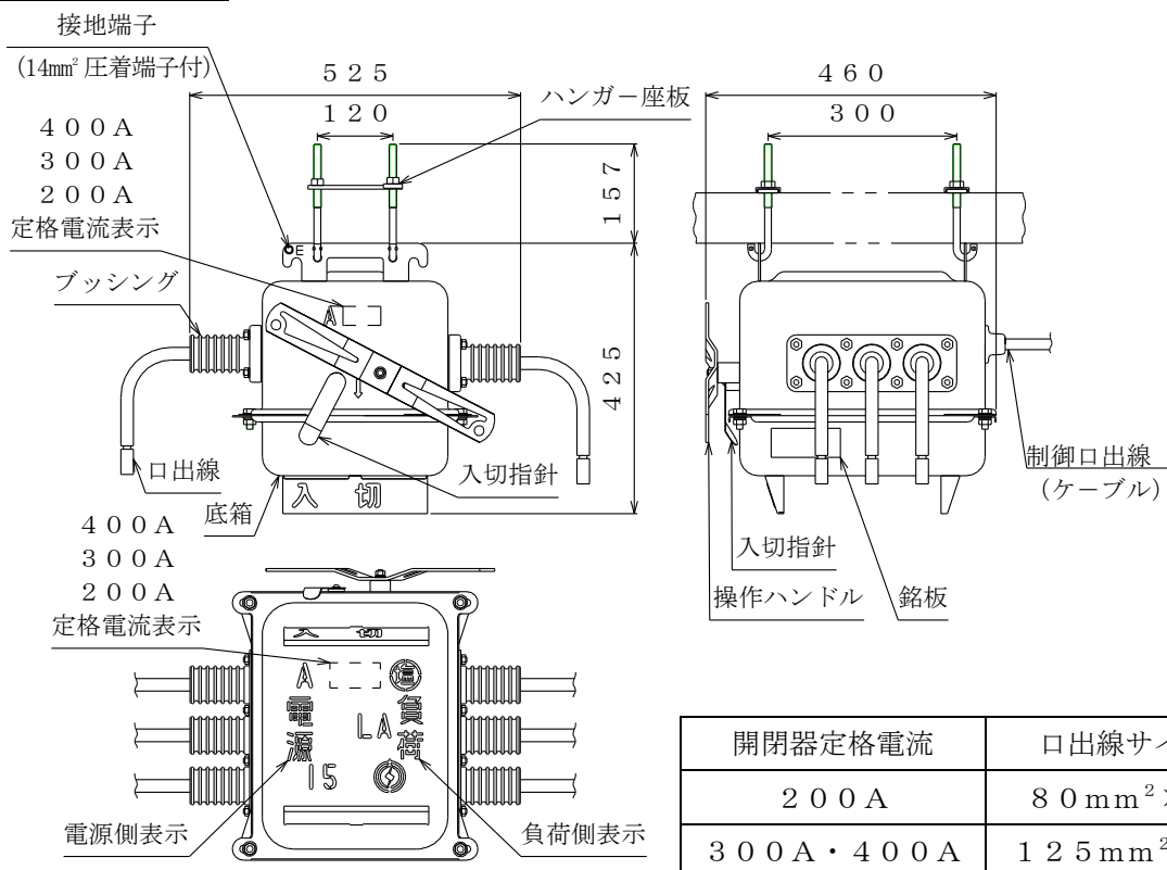
OAG-CLD5形高圧気中開閉器
