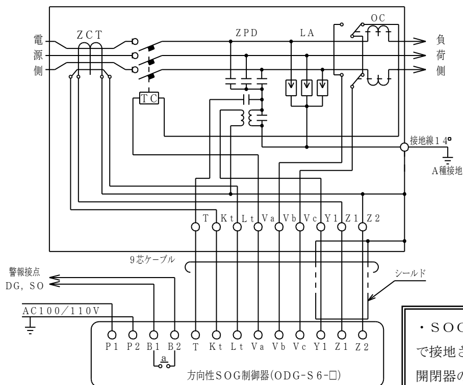
OAG-CLD5形高圧気中開閉器
