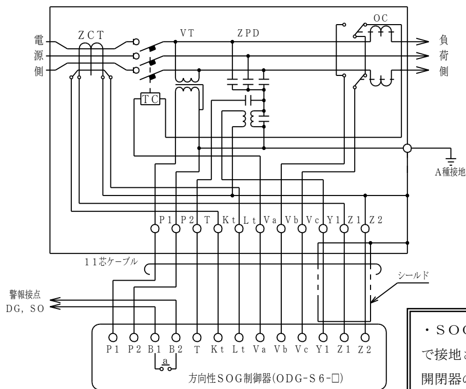
OAG-CPD5形高圧気中開閉器
