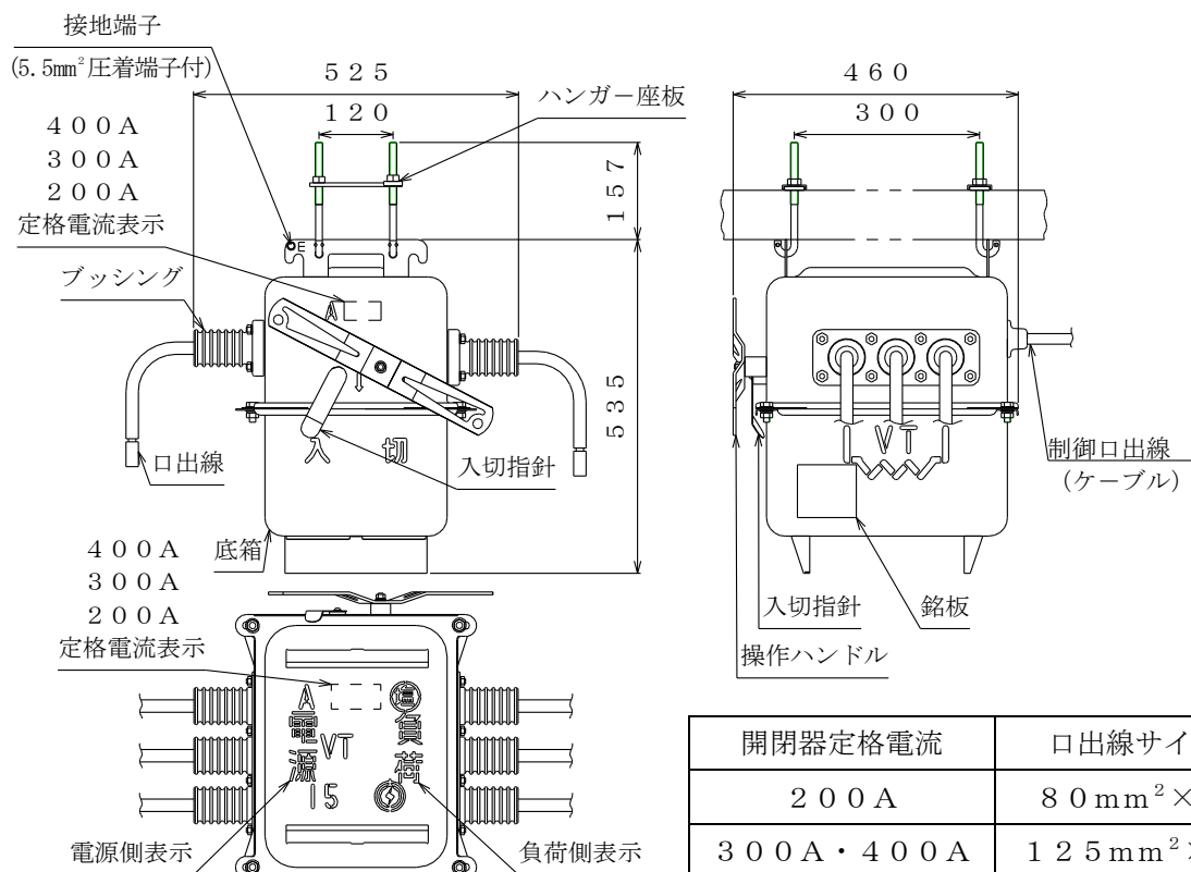
OAG-CPD5形高圧気中開閉器
