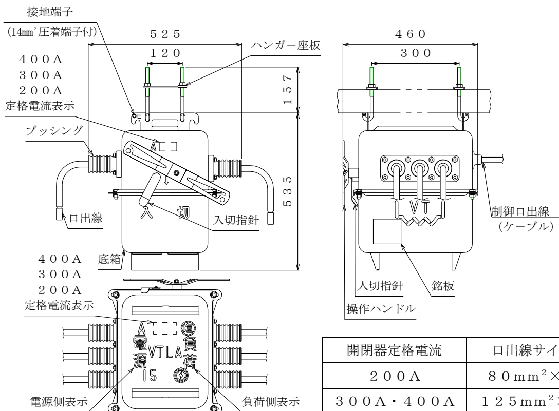
OAG-CPLD5形高压気中開閉器
