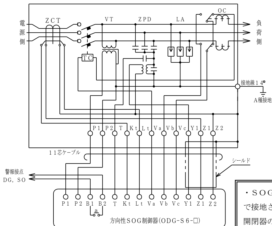
OAG-CPLD5形高压気中開閉器
