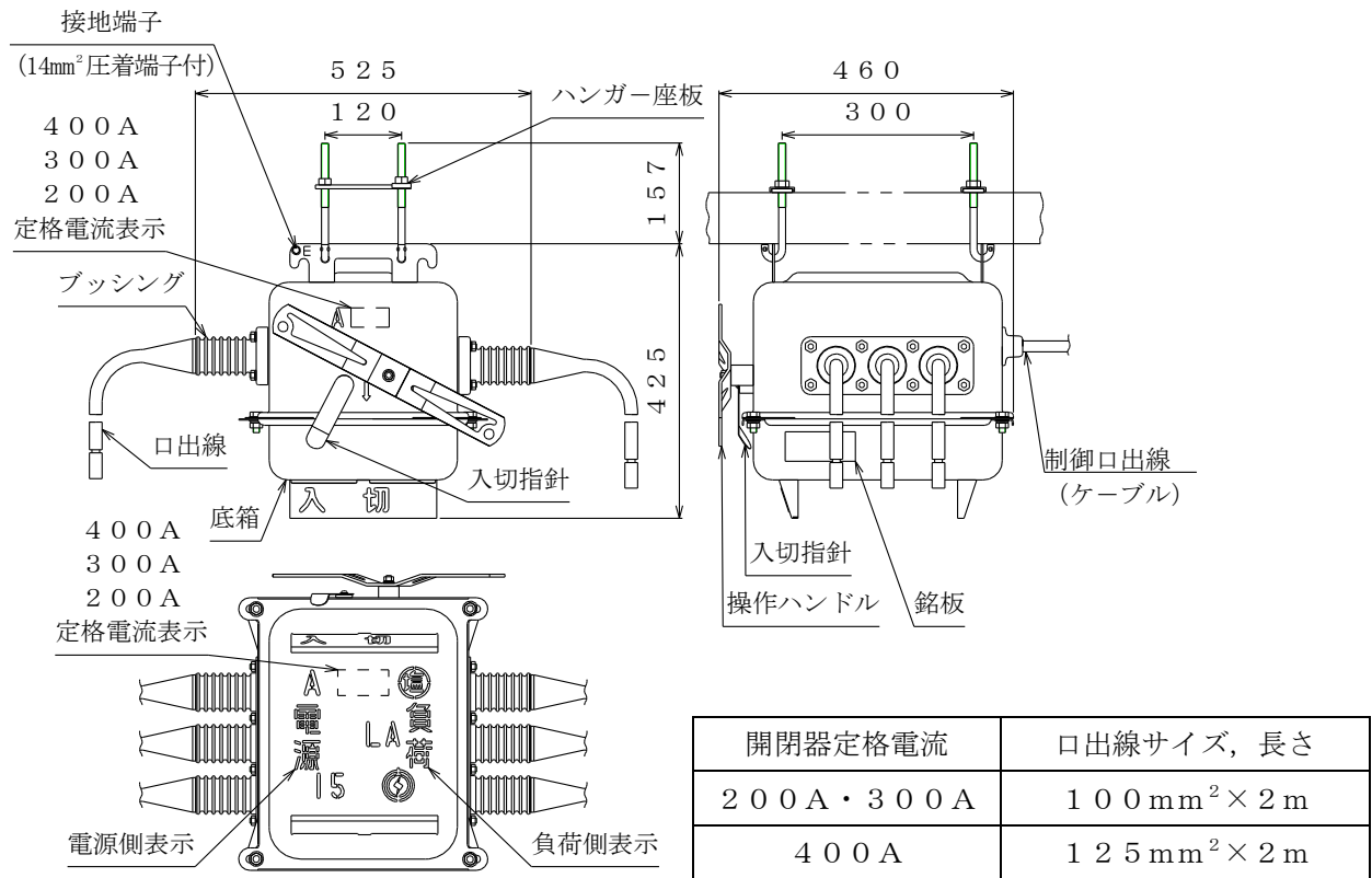
OAG-CLDK5形高圧気中開閉器
