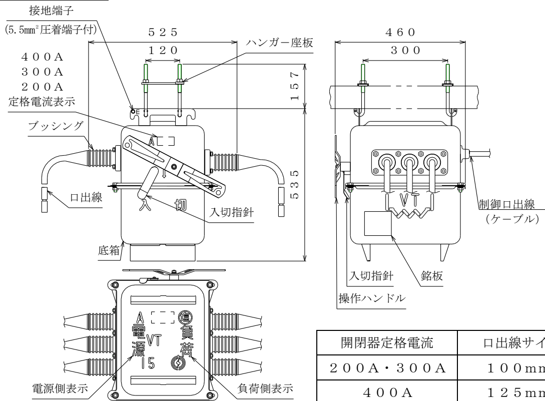
OAG-CPDK5形高圧気中開閉器
