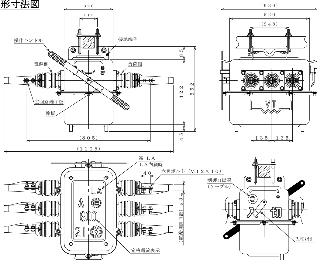
OAG-CPL6形高压気中開閉器
