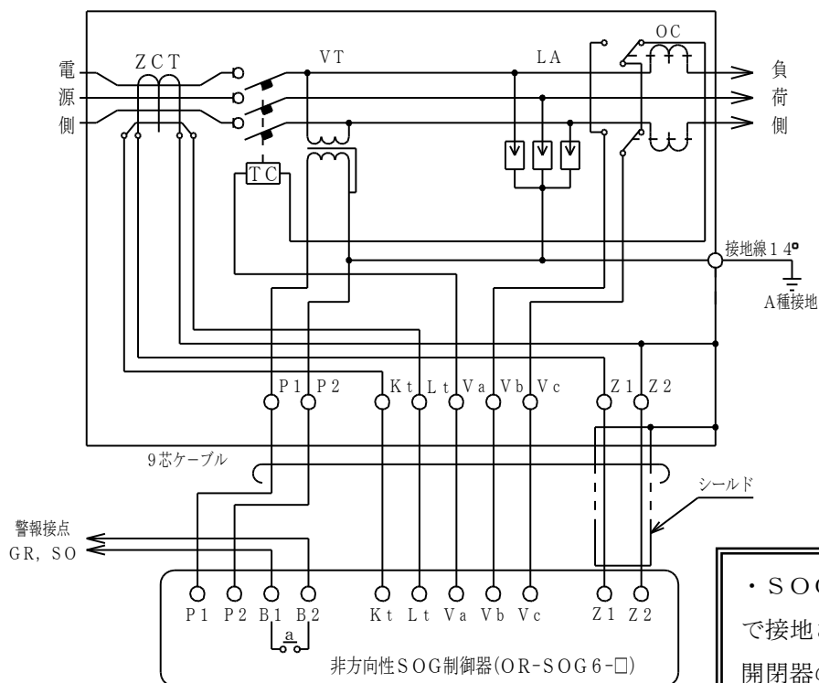
OAG-CPL6形高压気中開閉器
