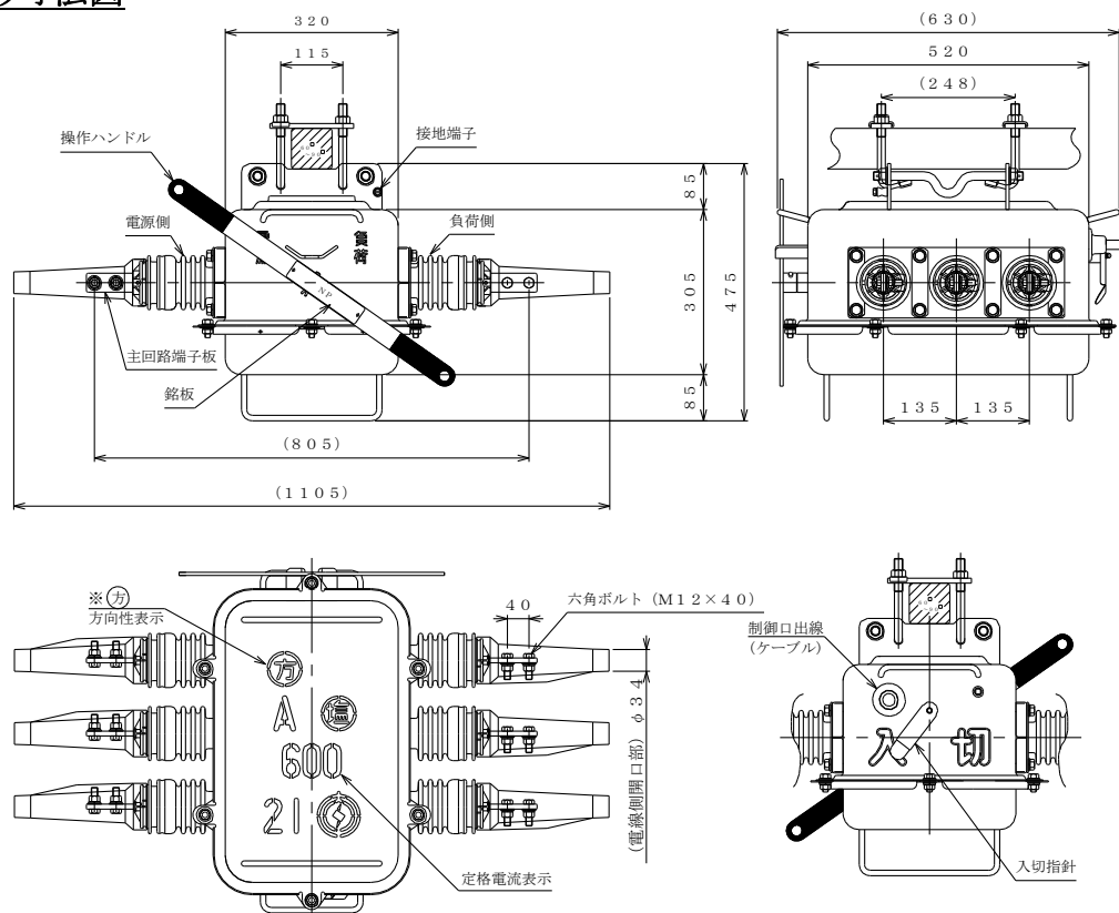
OAG-CD6形高圧気中開閉器
