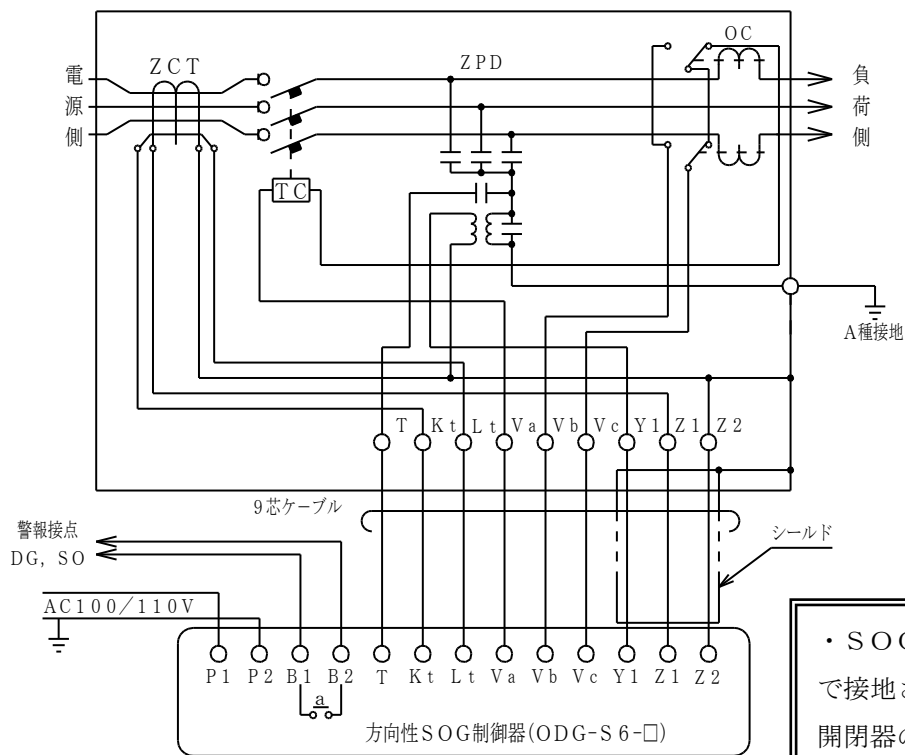
OAG-CD6形高圧気中開閉器
