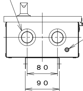
端子台符号詳細
