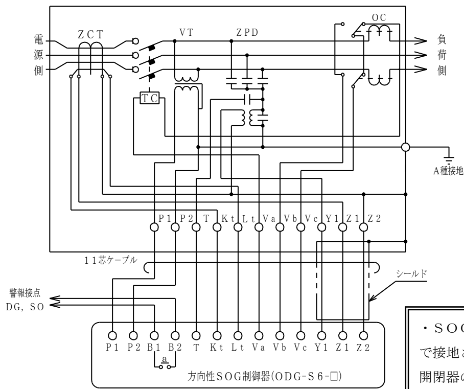
OAG-CPD 6 形高压気中開閉器
