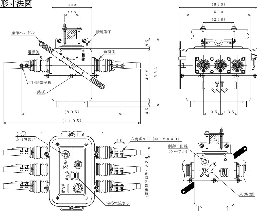
OAG-CPD 6 形高压気中開閉器
