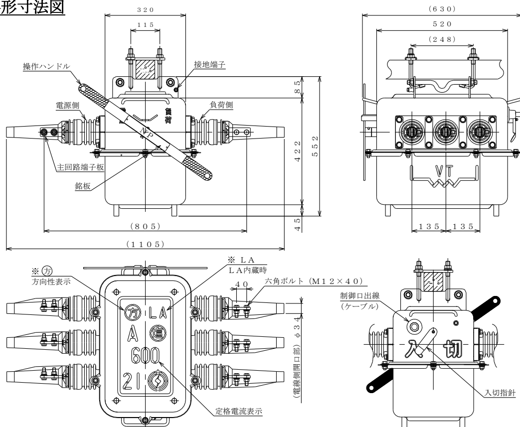
OAG-CPLD6形高压気中開閉器
