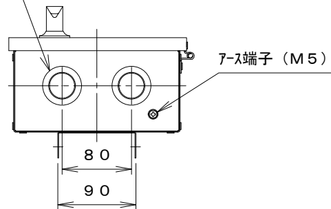
端子台符号詳細
