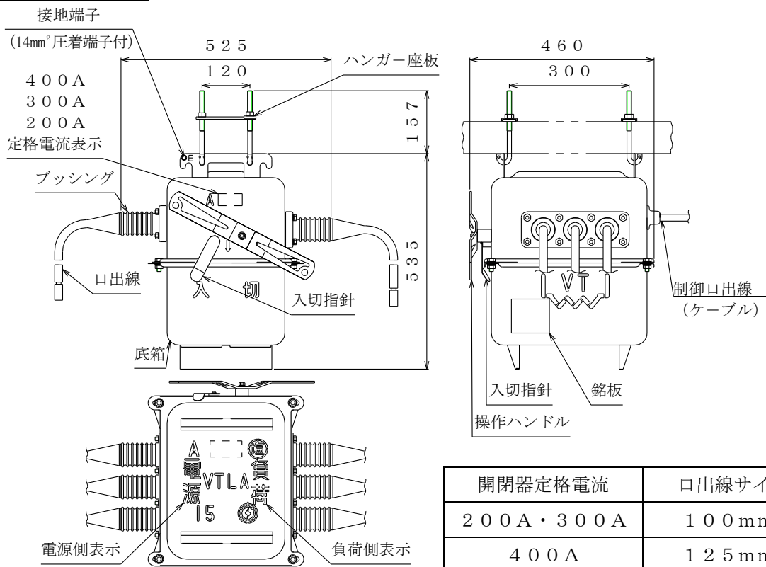
OAG-CPLK5形高圧気中開閉器
