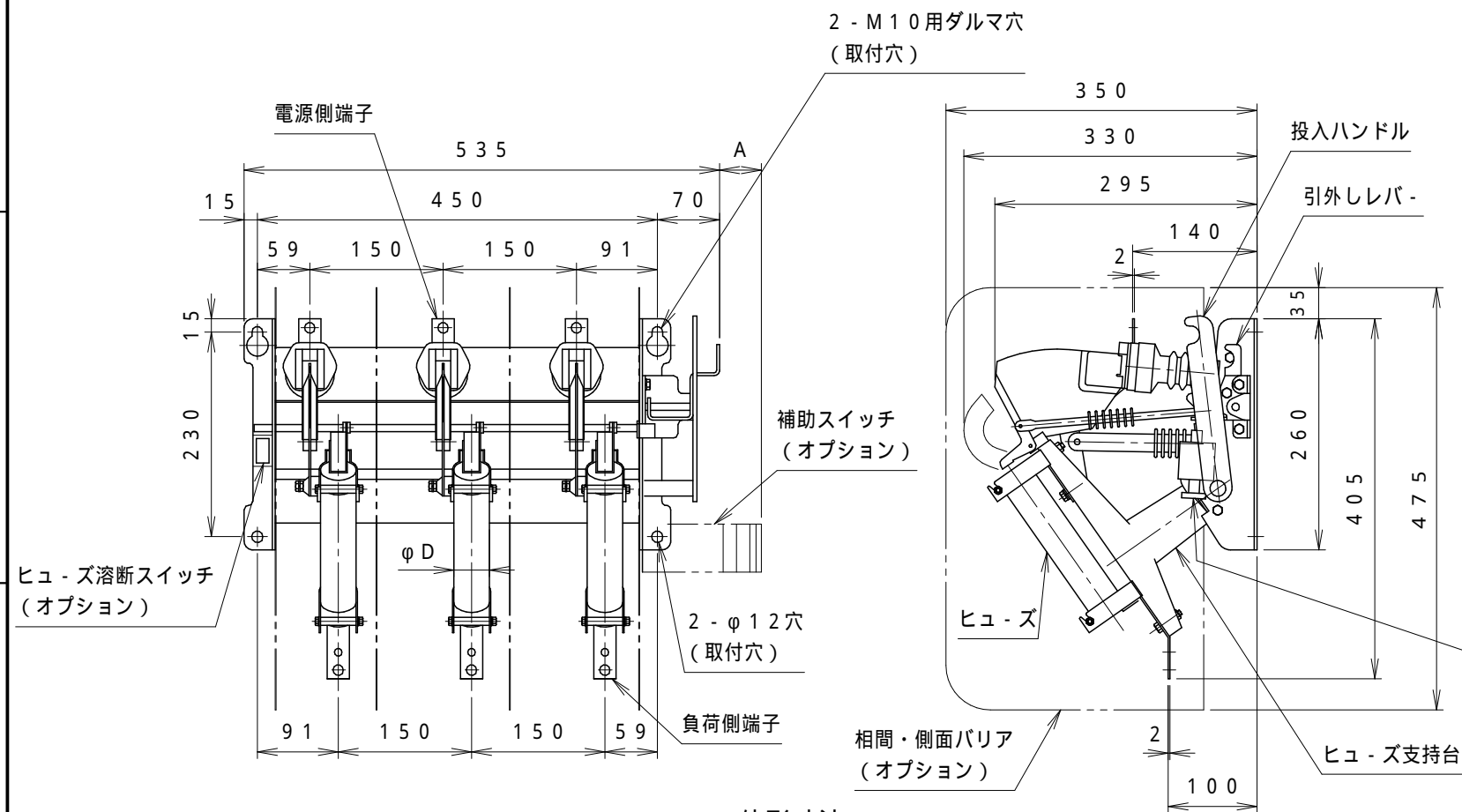
外形寸法
