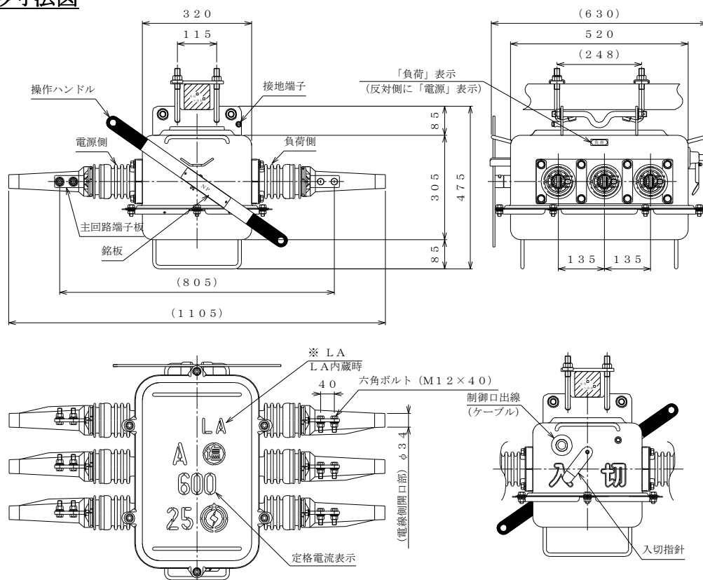
OAG-CL6形高压気中開閉器
