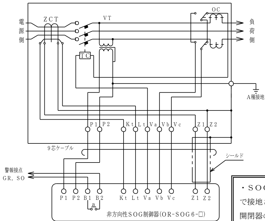
OAG-CP6形高圧気中開閉器
