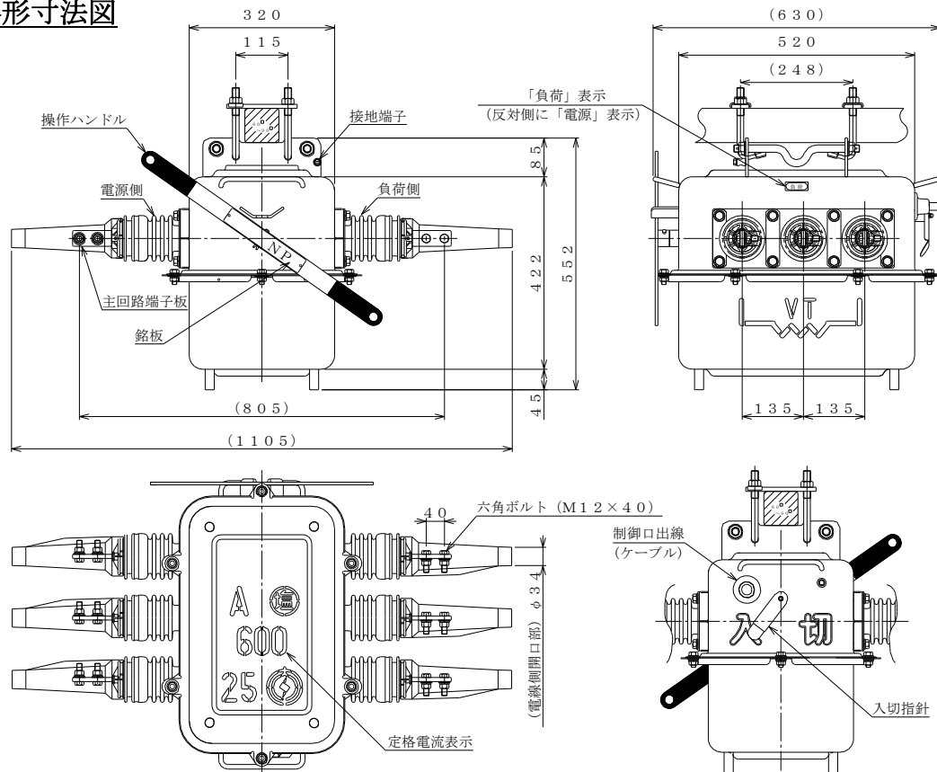
OAG-CP6形高圧気中開閉器
