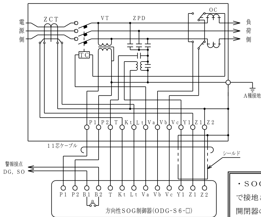
OAG-CPD 6 形高压気中開閉器
