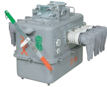
センサ内蔵自動気中開閉器 (長寿命形・スマートグリッド対応)
