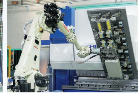
自動ベンディングシステム
